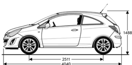
Seitenansicht 3 Türen Prospettiva laterale 3 porte
